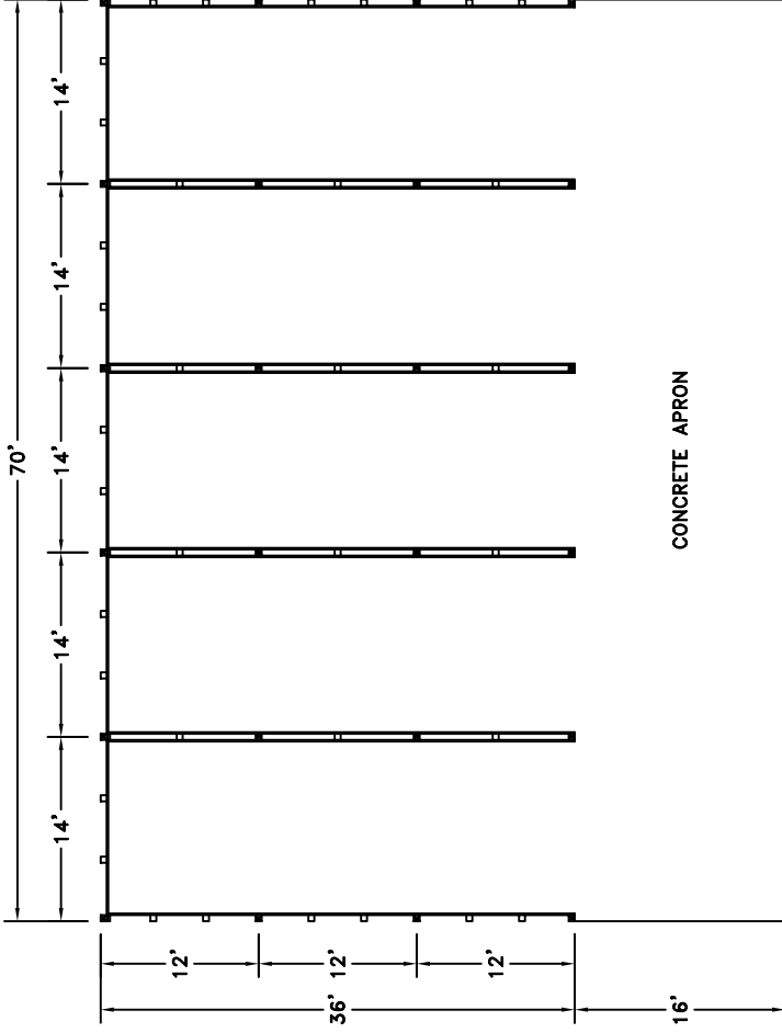
PLAN SCALE: 1/16"=1'-0"
