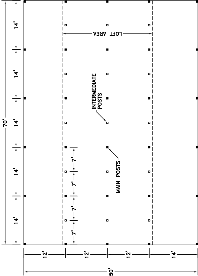
PLAN SCALE: 1/16"=1'-0"
