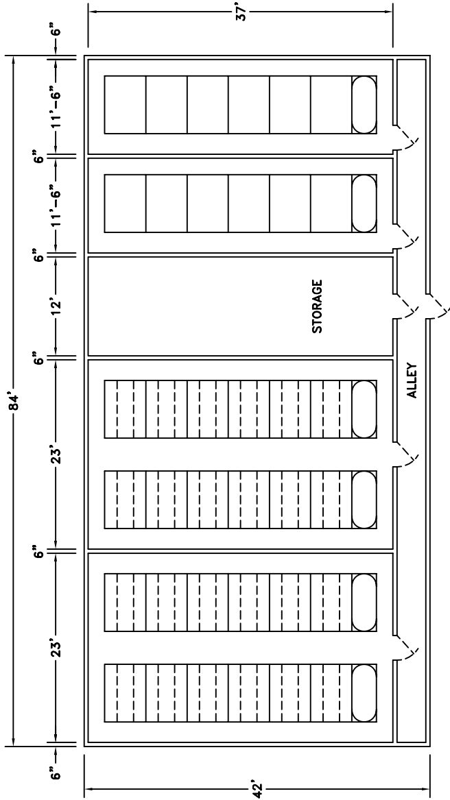
PLAN SCALE: 1/8"=1'-0"
