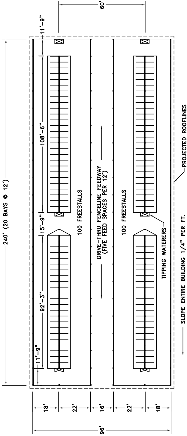
PLAN SCALE: 1"=40'
